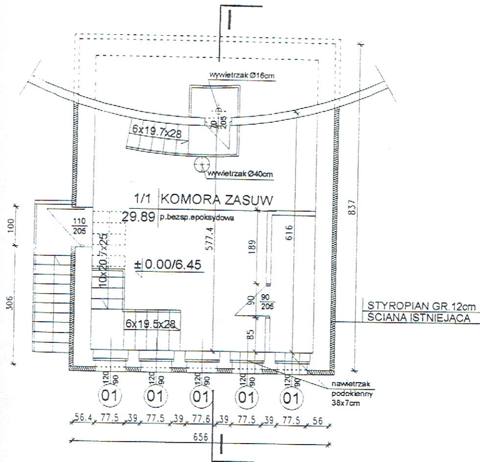
RZUT ±0.00 ZACH. 1:100
