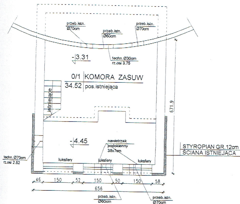
RZUT - 3.31 ZACH. 1:100
