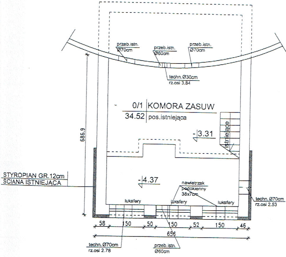
RZUT - 3.31 WSCH. 1:100
