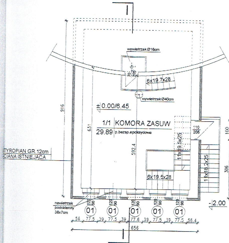
RZUT ±0.00 WSCH. 1:100
