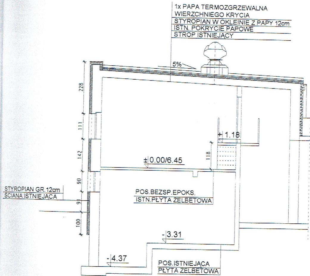
PRZEKRÓJ I-I WSCH. 1:100
